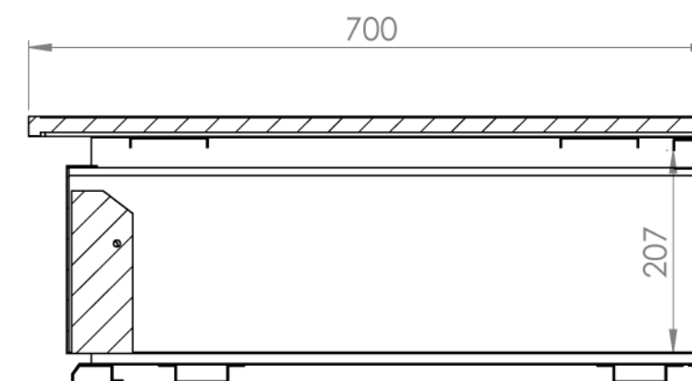
COUPE A-A ECHELLE 1 : 7
