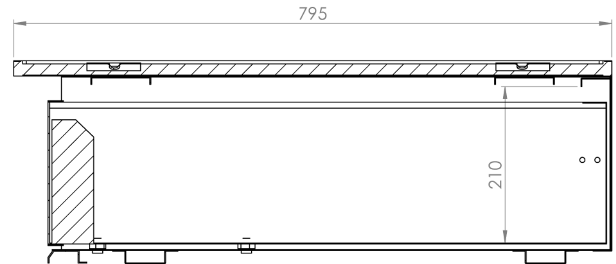
COUPE B-B ECHELLE 1 : 5
